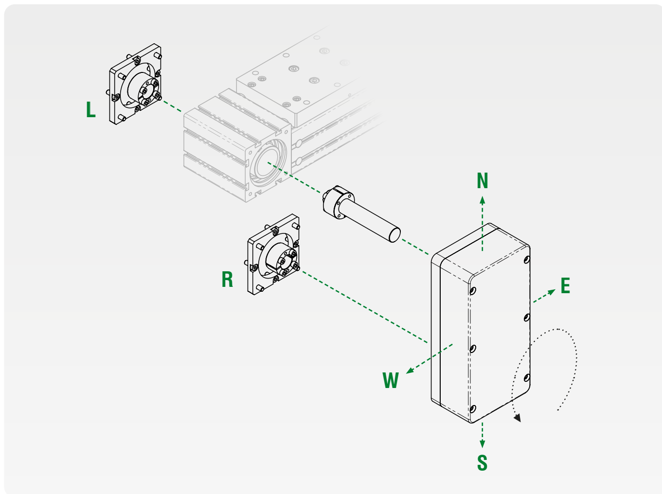
Flangia calettatore
