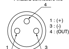
Pinatura connettore M8
