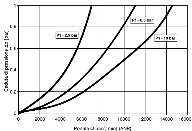
Curve di portata
