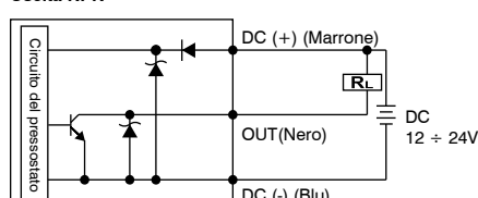
Uscita NPN
