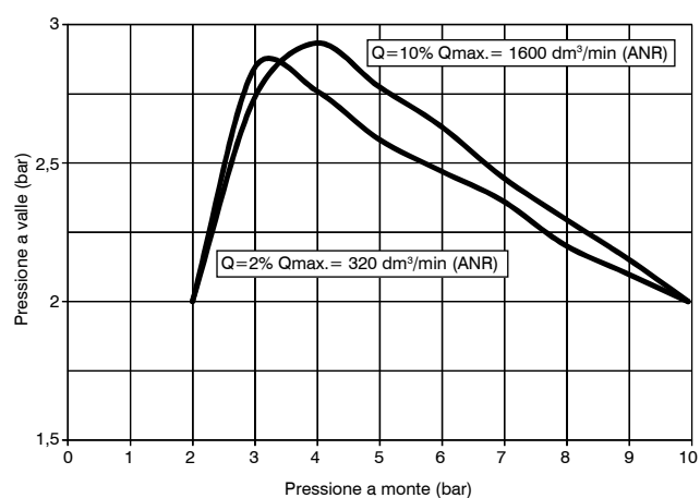
Caratteristica di regolazione
