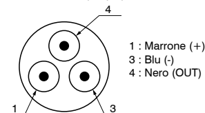
Pinatura cavo 3 fili
