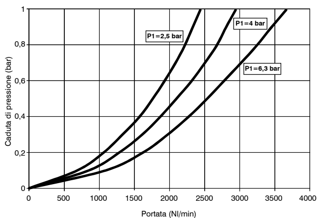
Curve di portata
