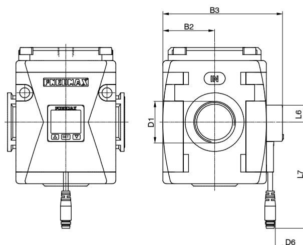
Versione con pressostato digitale incorporato
