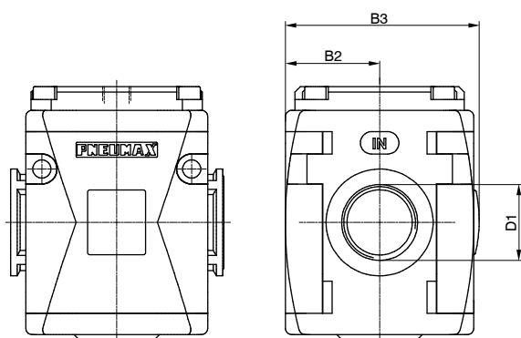
Versione con manometro incorporato
