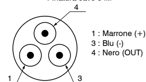
Pinatura cavo 3 fili
