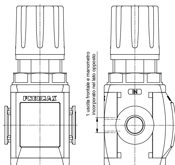
Versione con manometro incorporato
