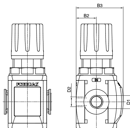
Versione con manometro incorporato (M)
