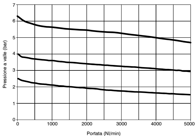
TG4 - G1" 0-8 bar P1=10 bar
