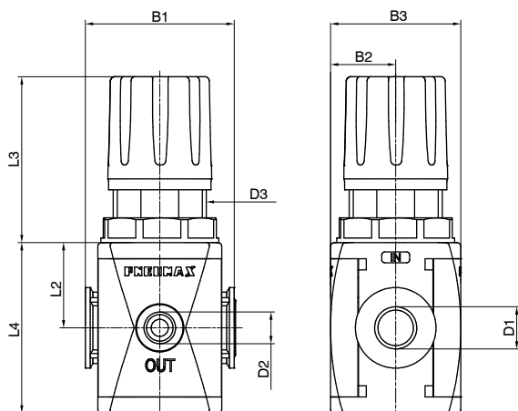
Versione con presa manometro (B)
