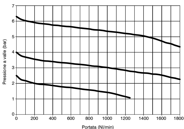
TG2 - G3/8" 0-8 bar P1=7 bar
