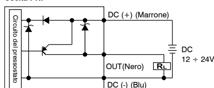
Uscita PNP
