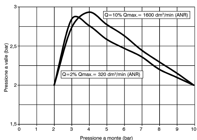
Caratteristica di regolazione
